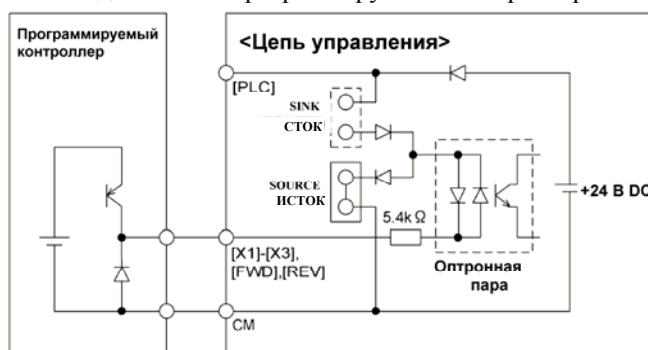
Рис. 2.16 (b). Подключение программируемого контроллера
