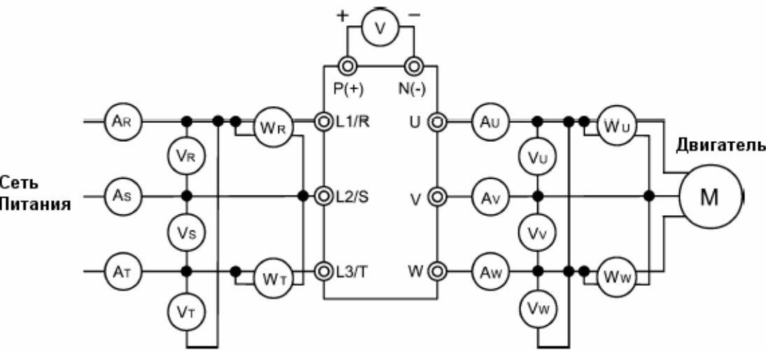
Рис. 7.1. Подключение измерительных приборов
