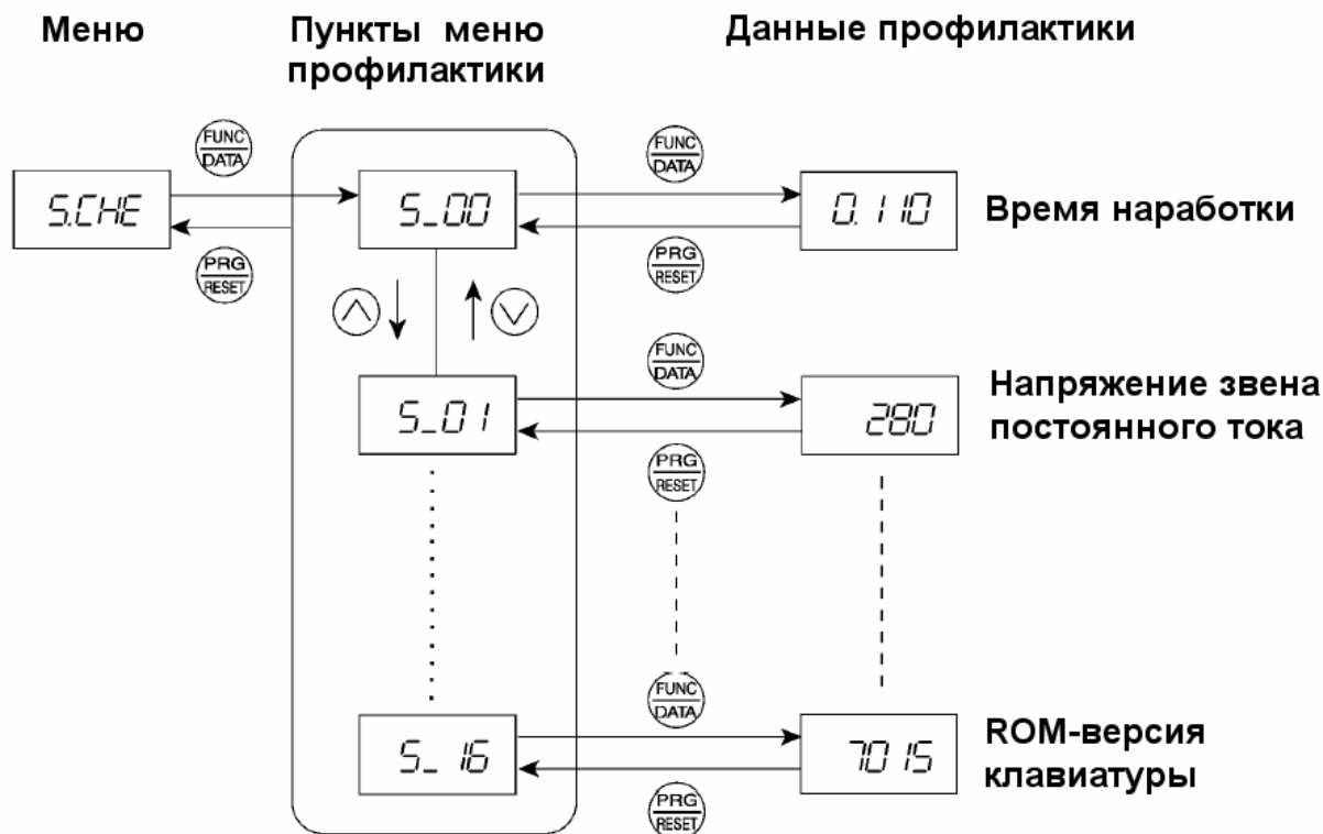
Рис.3.9. Переходы состояний в Меню "Профилактические данные"
