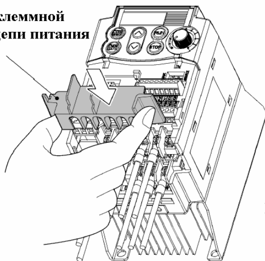
Рис. 2.11. Установка на место крышки КК цепи питания.
