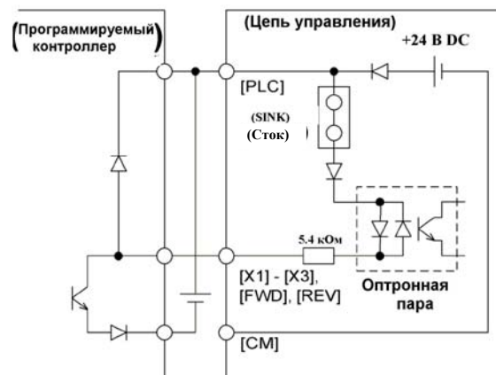
Рис. 2.15. Подключение внешнего питания
