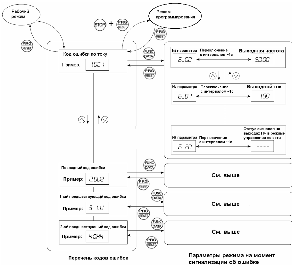
Рис. 3.2. Переход состояний в аварийном режиме
