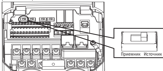
Рисунок 4.4.1. Переключатель «приемник/источник»
