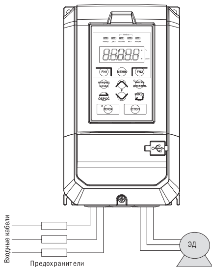
Рисунок 3.4. Установка плавких предохранителей
