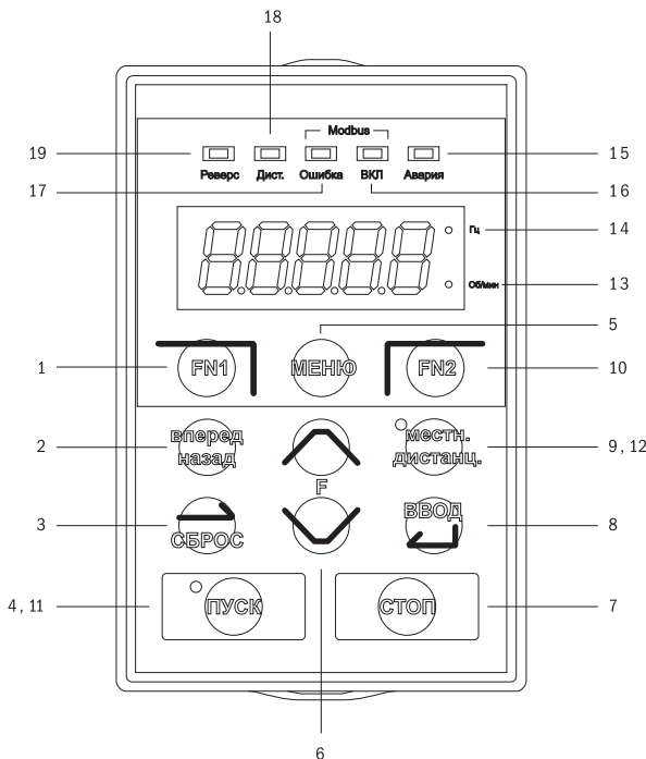
Рисунок 5.1.1.1. Кнопочная панель
