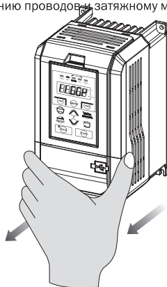
Шаг 2. Снимите крышку клеммной коробки
