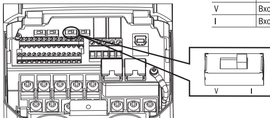
Рисунок 4.4.2. Переключатель A2
