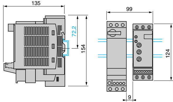
Система TeSys модели U (силовой модуль с одним или двумя направлениями вращения) и ATSU 01N206LT - ATSU 01N212LT Установка вплотную друг к другу
