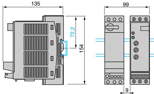
Система TeSys модели U (силовой модуль с одним или двумя направлениями вращения) и ATSU 01N222LT - ATSU 01N232LT Установка вплотную друг к другу
